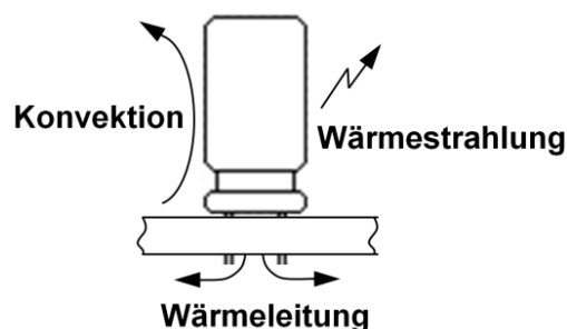
Abb. 4: Kühlungsmechanismen von Elkos
