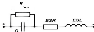
Abb. 2: Ersatzschaltbild des Elektrolytkondensators
