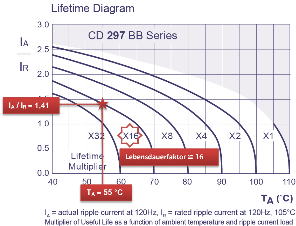
Abb. 9: Der Schnittpunkt der Betriebspunktparameter führt zum Lebensdauerfaktor
