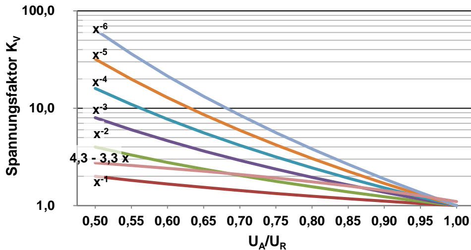
Abb. 8: Spannungsfaktoren verschiedener Hersteller im Vergleich [4]
