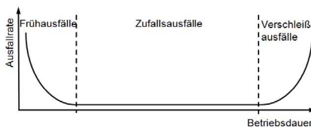
Abb. 6: Zeitliche Entwicklung der Ausfallrate
