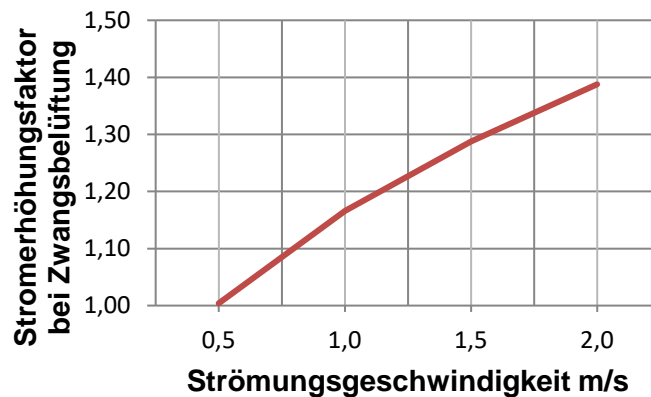
Abb. 5: Erhöhung der Strombelastbarkeit durch Zwangskühlung
