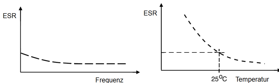
Abb. 3: (a) Frequenz- und (b) Temperaturabhängigkeit des ESR
