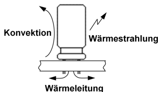
Abb. 4: Kühlungsmechanismen von Elkos
