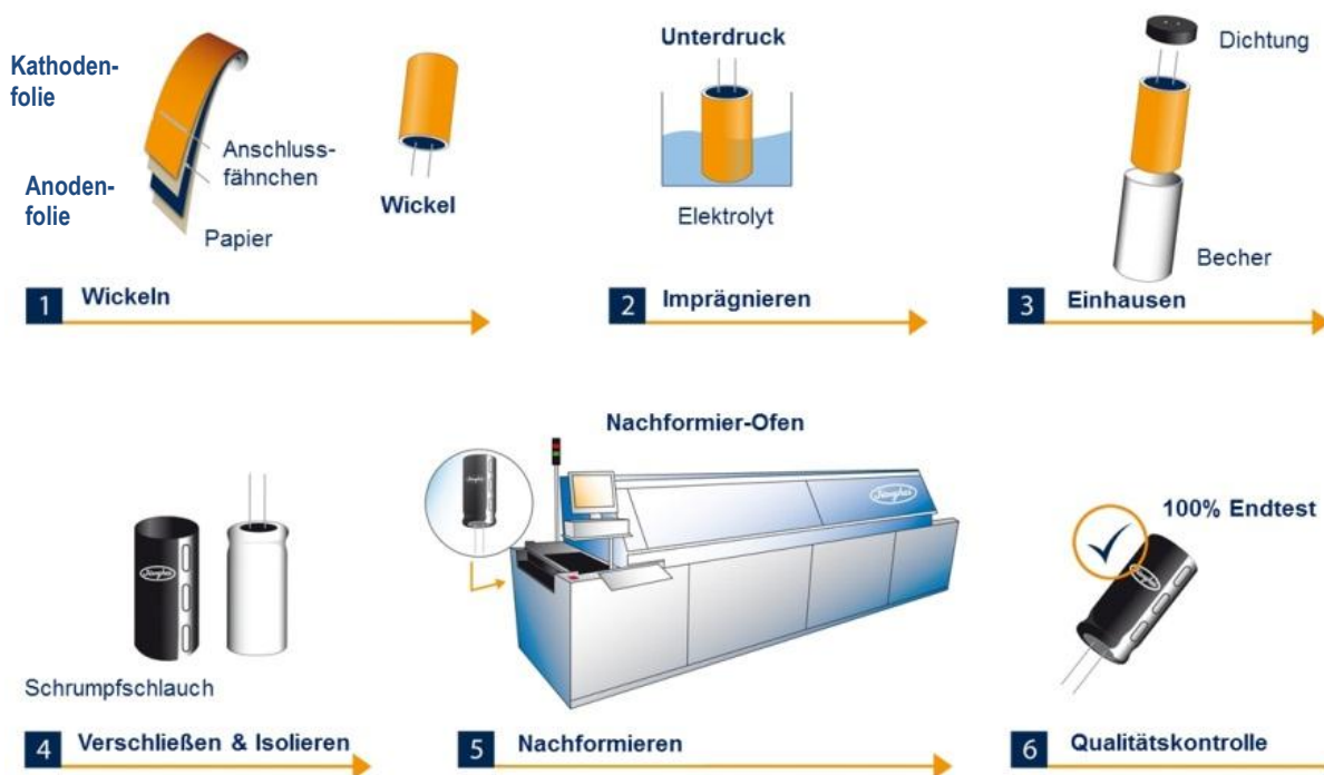
Abb. 3: Prozessschritte vom Vormaterial zum Elko
