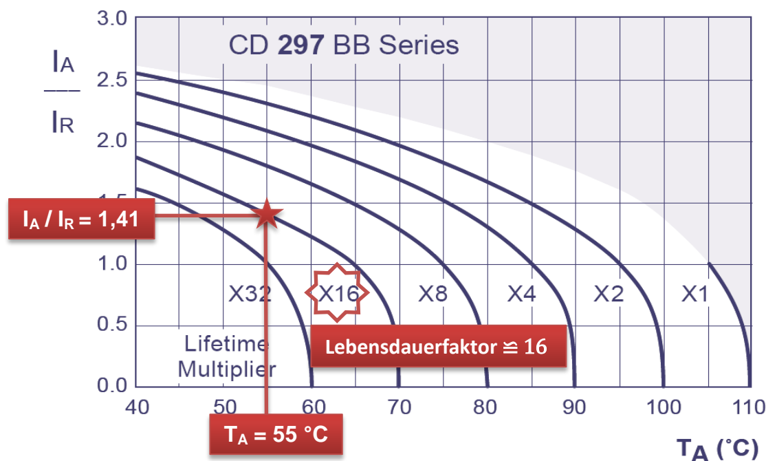
Abb. 9: Der Schnittpunkt der Betriebspunktparameter führt zum Lebensdauerfaktor
