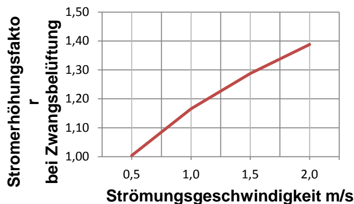
Abb. 5: Erhöhung der Strombelastbarkeit durch Zwangskühlung
